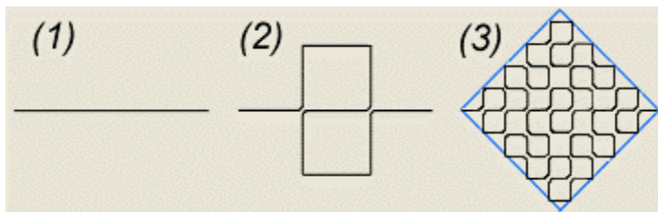
Curva de Peano
